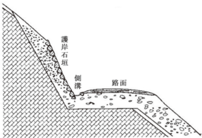
明治の道路の断面図模式図
